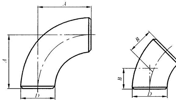
图 1 长半径弯头
