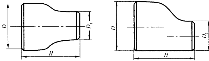
图 10 异径接头
