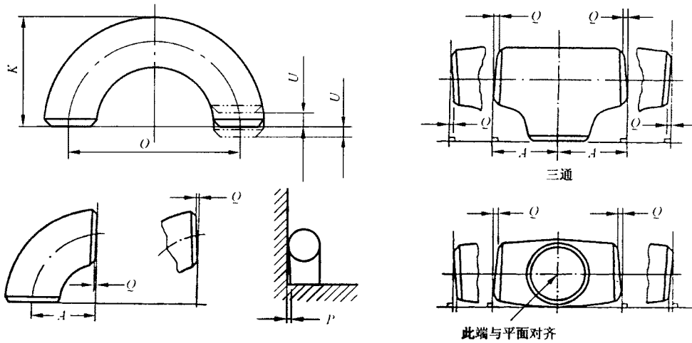
图 11 公差简图
