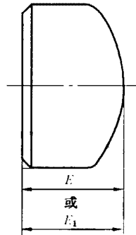
图 A.10 管帽
