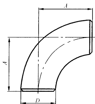
图 4 短半径弯头
